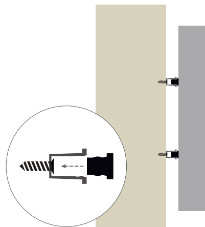
C OPCIÓN INSTALACIÓN: Separadores macho-hembra
