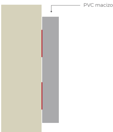
A OPCIÓN INSTALACIÓN: Polímero / adhesivo
