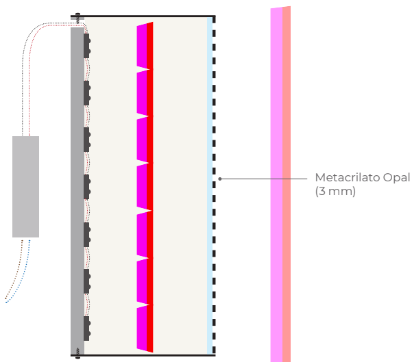
A OPCIÓN FRENTE: Metacrilato Opal 3 mm
